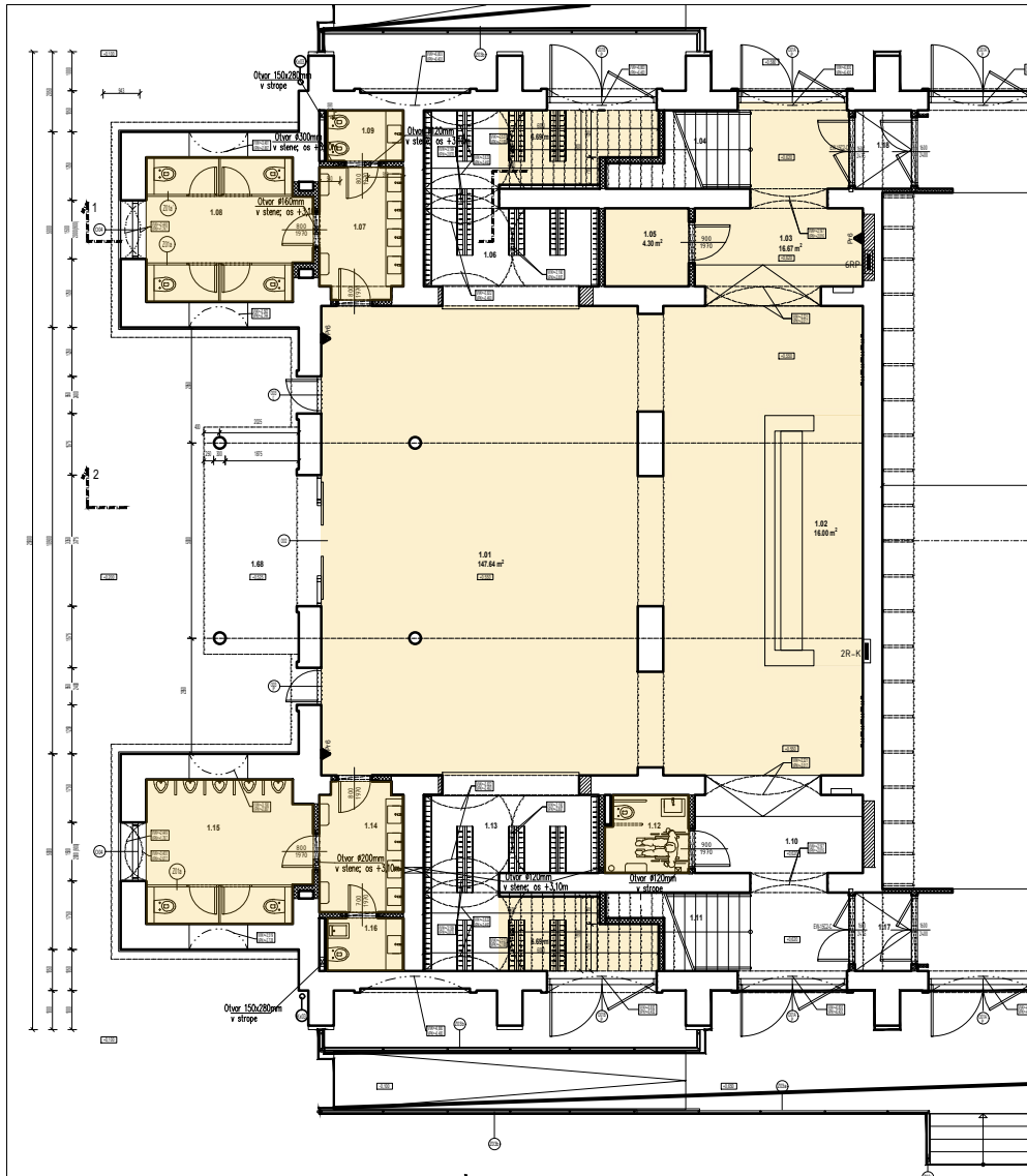
Pôdorys 1.NP
