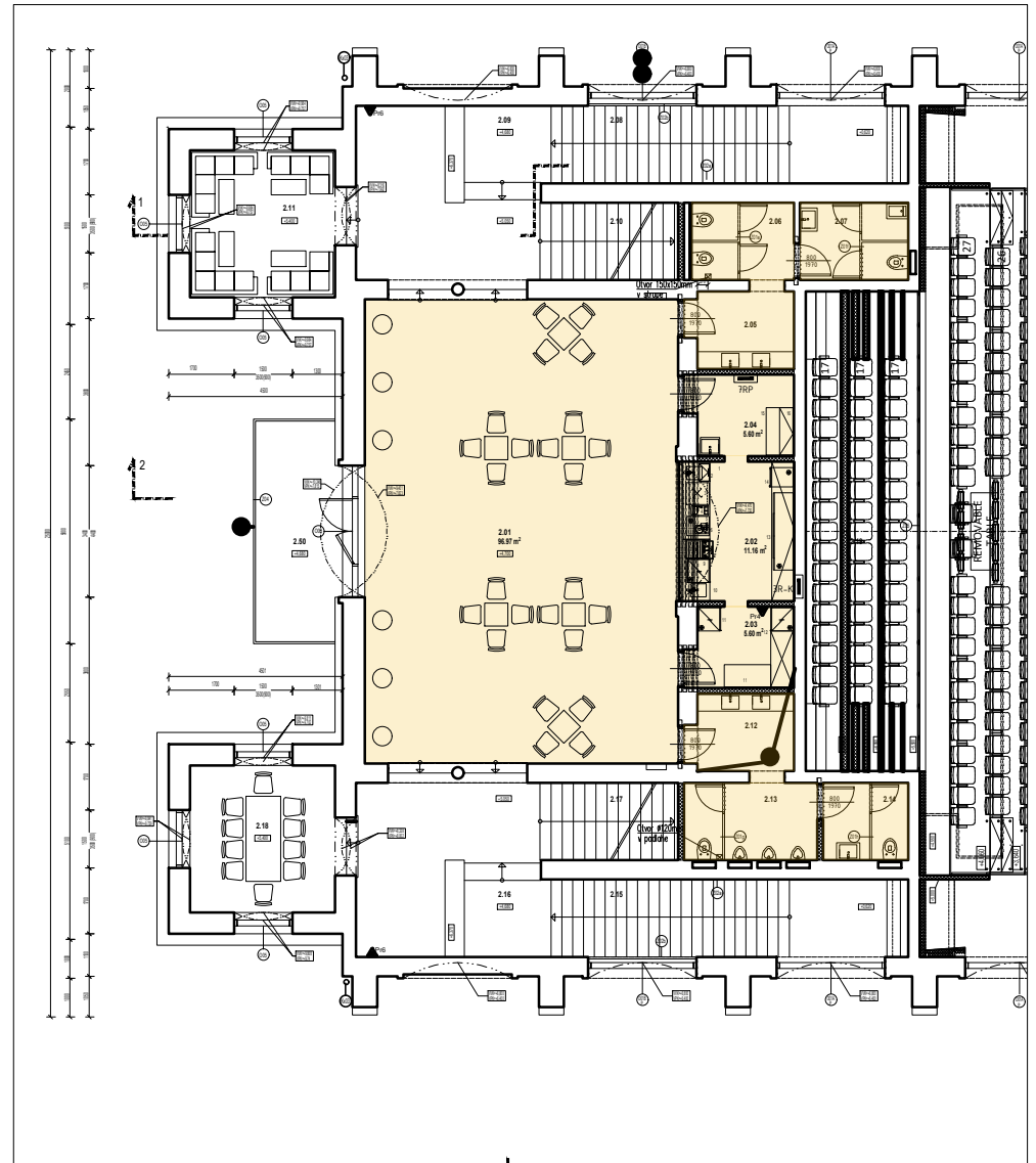
Pôdorys 2.NP
